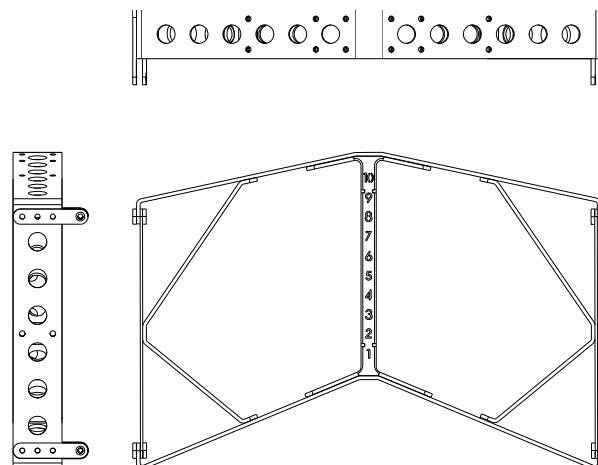
Fig.28. TA-X210R Frame
