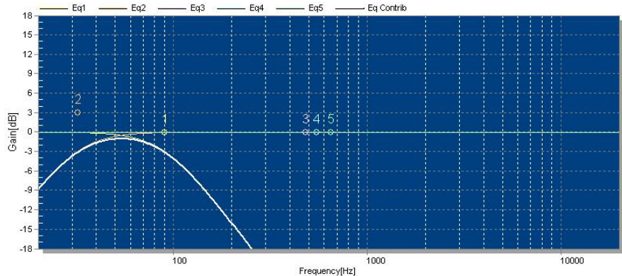
Fig.18. X218W3K PRESET options
